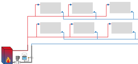
Afb. 9.52 Tichelman systeem (tweepijpssysteem, aanvoerleiding en retourleiding van en naar alle radiatoren even lang)
