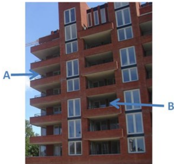
Afb. 16.8 Raam A heeft een overstek en een zijbelemmering, raam B heeft een overstek en twee zijbelemmeringen
