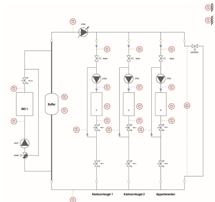
Afb. 9.63 Buffervat in het hydraulisch prinscipeschema naast warmteopwrekker WO1
