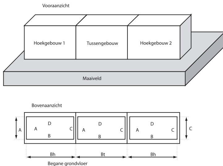
Afb. 8.19 Perimeter bij hoek- en tussengebouwen
