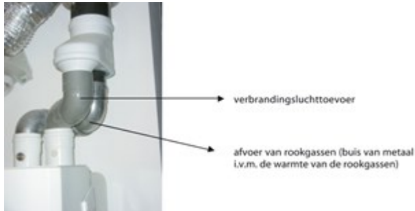
Afb. 9.15 Gesloten toestel met aansluiting van verbrandingsluchttoevoer en rookgasafvoer
