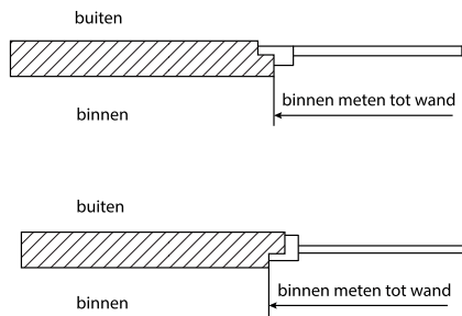
Afb. 8.14 Kozijnwerk binnenmaat
