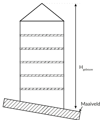
Afb. 7.10 Bepalen van de gebouwhoogte
