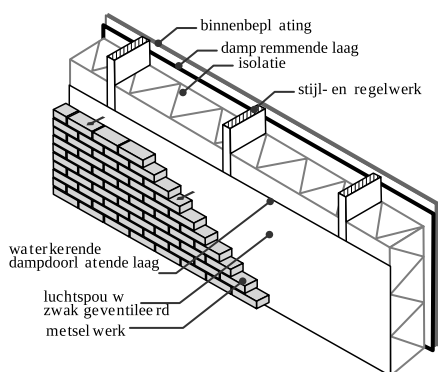
Afb. 8.28 Spouwconstructie
