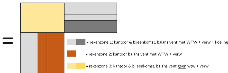
Afb. 6.4 Voorbeeld van de indeling van het gebouw – stap 4
