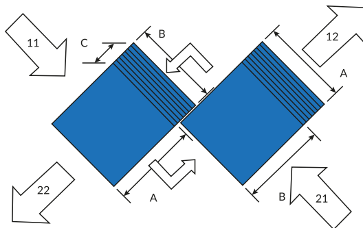
Afb. 11.43 Schematische voorstelling van een dubbele kruisstroomwarmtewisselaar
