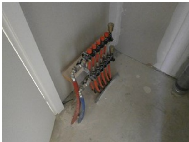
Afb. 9.59 Verdeler/verzamelaar
