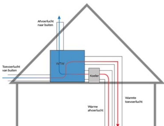
Afb. 10.22 Dauwpuntskoeling op ventilatielucht
