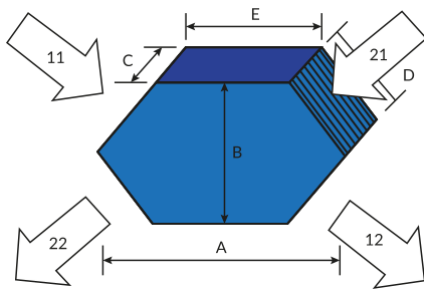
Afb. 11.49 Tegenstroomwarmtewisselaar
